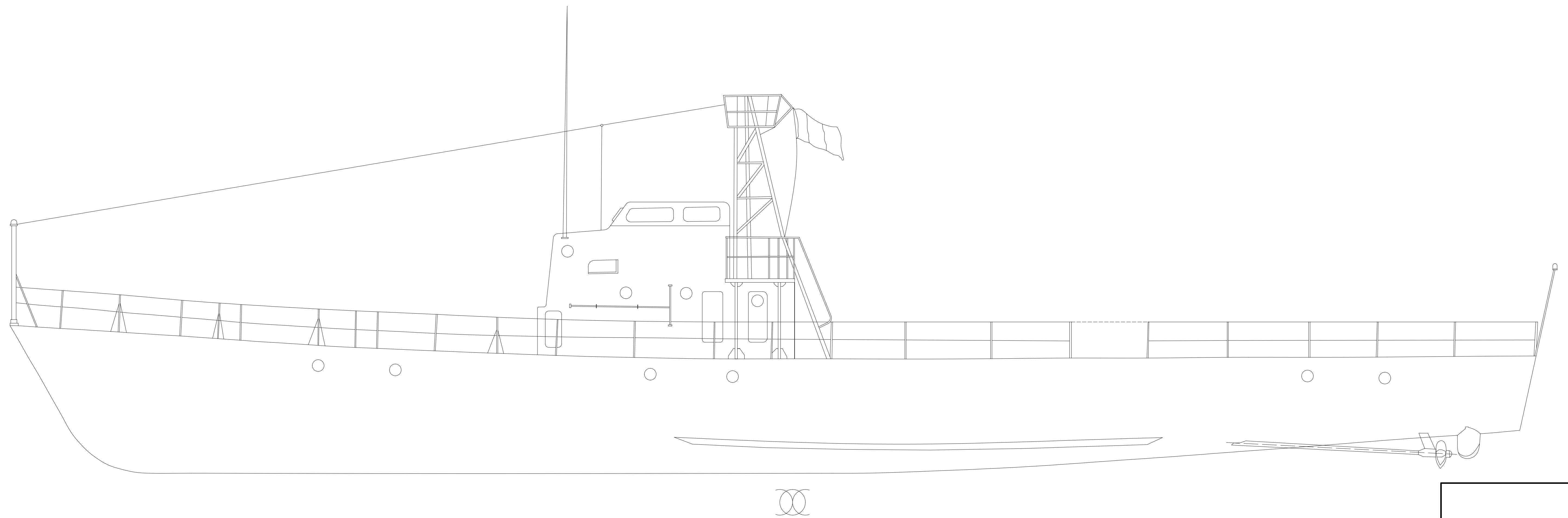
VEDERE LATERALA - EST SCARA 1/50
